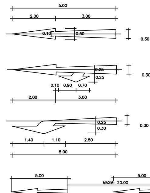
MARKA UNTUK PENYEBERANGAN PEJALAN KAKI
