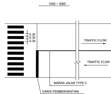
MARKA UNTUK PENYEBERANGAN PEJALAN KAKI
