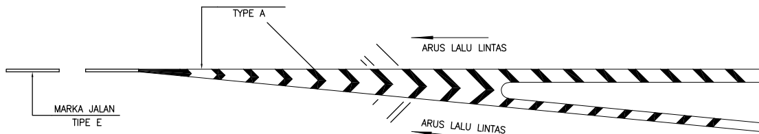
MARKA JALAN PADA UJUNG PENGGABUNGAN SKALA 1 : 100
