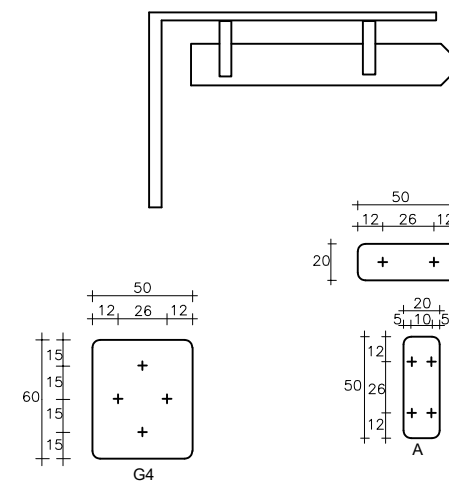
UKURAN RAMBU DAN PENEMPATAN BAUT N.T.S
