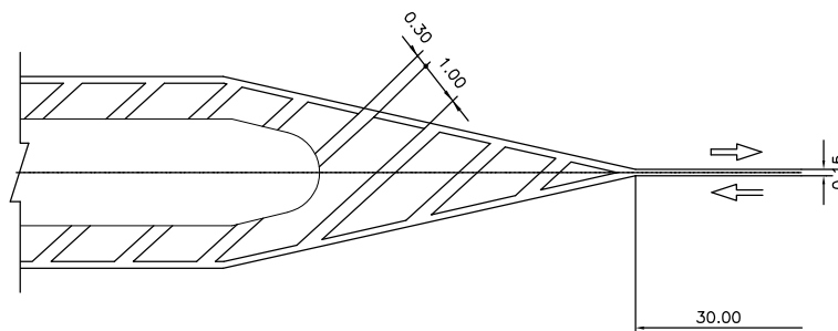
MARKA JALAN PADA PEMBUKAAN MEDIAN SKALA 1 : 100
