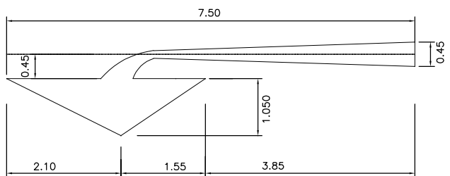
TIPE 3 SKALA 1 : 50
