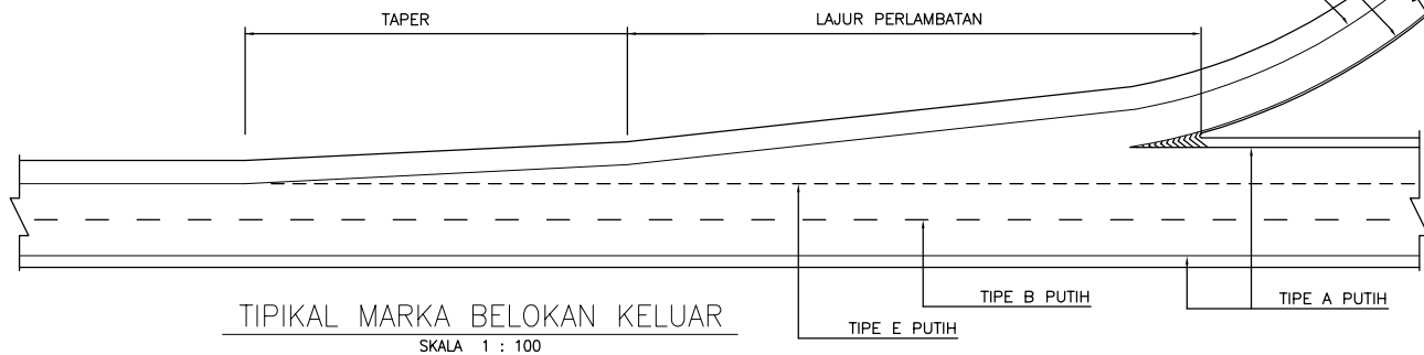
TIPE MARKA LAJUR
