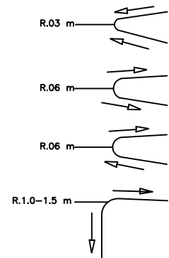
RADIUS UJUNG PULAU
