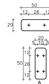
UKURAN RAMBU DAN PENEMPATAN BAUT N.T.S
